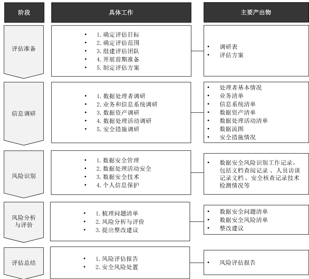
图 3 数据安全风险评估实施流程图
